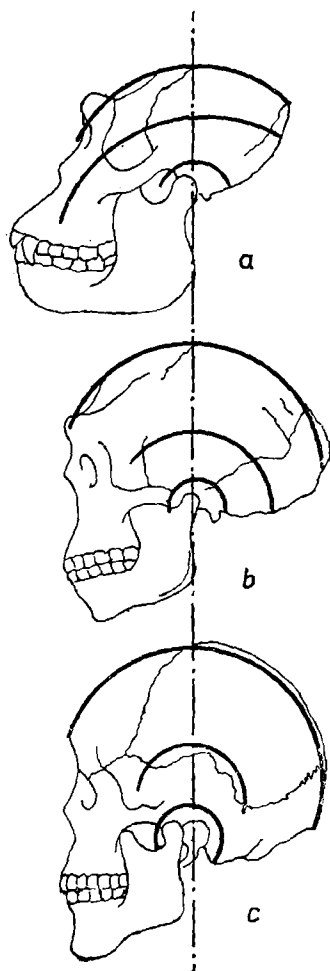
6. ábra. – Az emberi koponya begöngyölődése, az Anthropoidáktól kezdve. (Weidenreich után) a: Gorilla b: Sinanthropus c: Modern Ember
