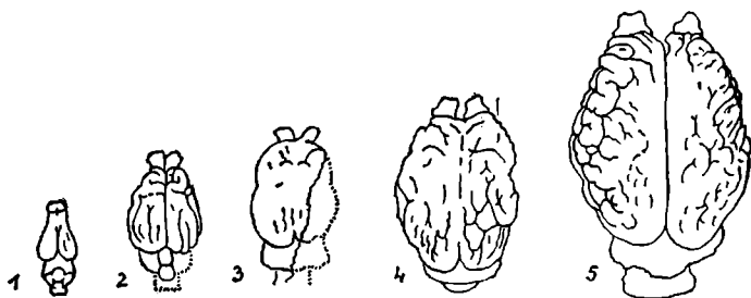
4. ábra. – Az agy fejlődése a Lóféléknél (Edinger után).
