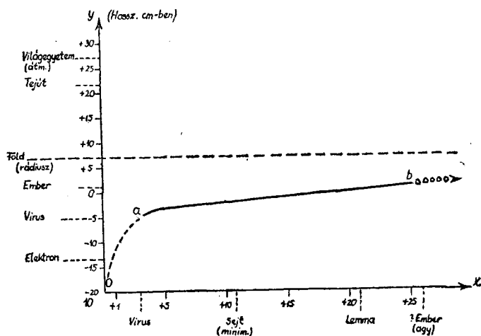
1. ábra. – A Komplexitások természetes görbéje. (l. a szöveget.)
