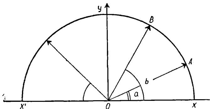
3. ábra. – A „cerebráció hullámának” szimbólikus kifejezése.
