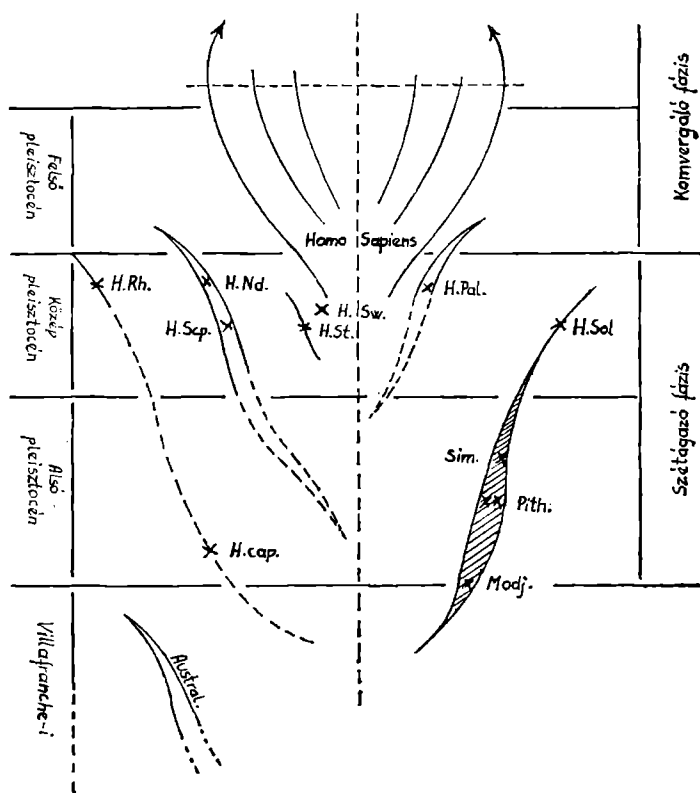
5. ábra. – Az Emberfélék kévéje.
