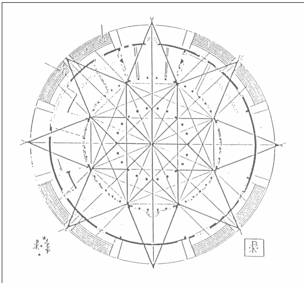
„Mennyei geometria” – A Santo Stefano Rotondo alaprajza
